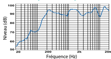
Réponse en fréquence
