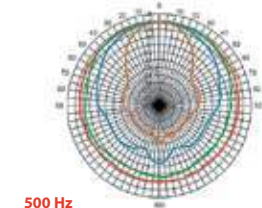
Directivité verticale
