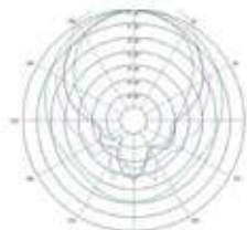
Directivité verticale
