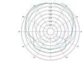
Directivité verticale
