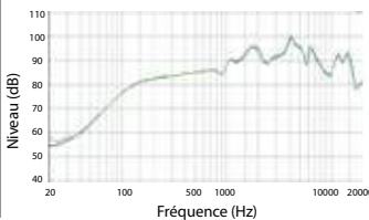
Bande passante
