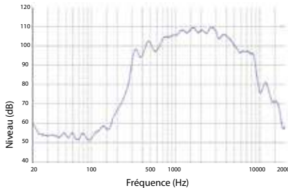
Bande passante
