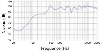
Bande passante
