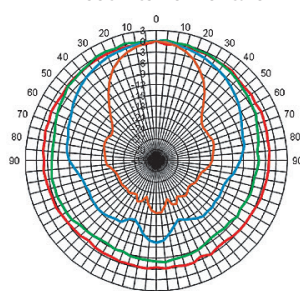
Directivité horizontale
