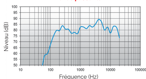
Bande passante
