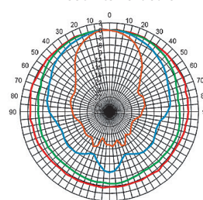
Directivité verticale
