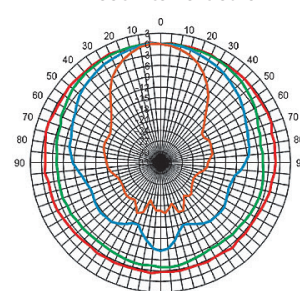
Directivité verticale
