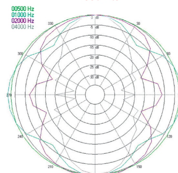
Directivité
