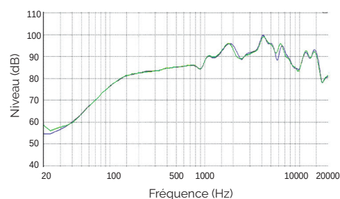
Bande passante
